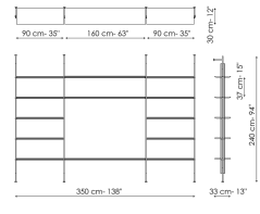
Wall fixing tv-stand module Width: 350cm Depth: 33cm Height: 240cm
