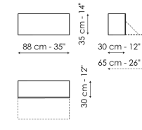
Box Width: 88cm Depth: 30cm Height: 35cm
